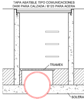
ALZADO
